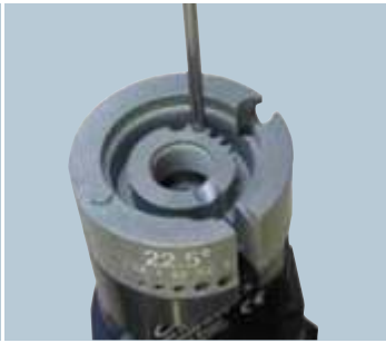
Refrentado de electrodos
